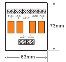
ILM-200 Interlock Module
